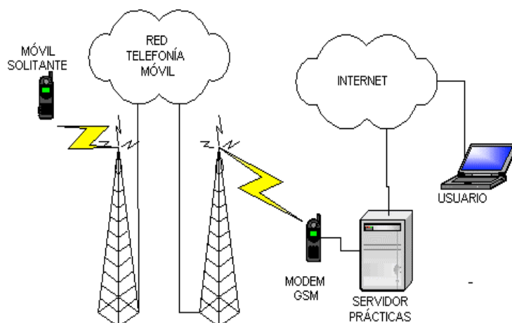
Figura 3. Esquema y funcionamiento del sistema
